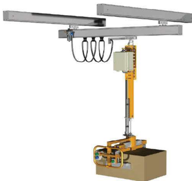
剛性提昇機
