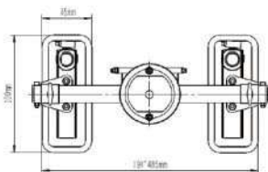
雙腳吸盤85x200mm，吸力50Kg。 訂貨號812450
