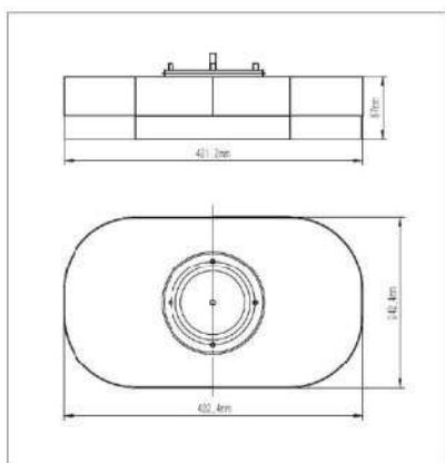
塑殼吸盤240x420mm。訂貨號816420
